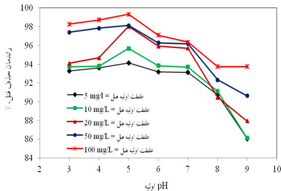
نمودار ۱- اثر pH اولیه محلول بر راندمان حذف در غلظت‌های مختلف فنل (غلظت منعقدکننده معادل ۰/۱ ml/L)
