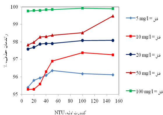
نمودار ۳- اثر کدورت اولیه بر راندمان حذف فنل از محلول سنتتیک، در غلظت‌های مختلف (pH برابر ۵، غلظت منعقدکننده برابر ۰/۱ ml/L)
