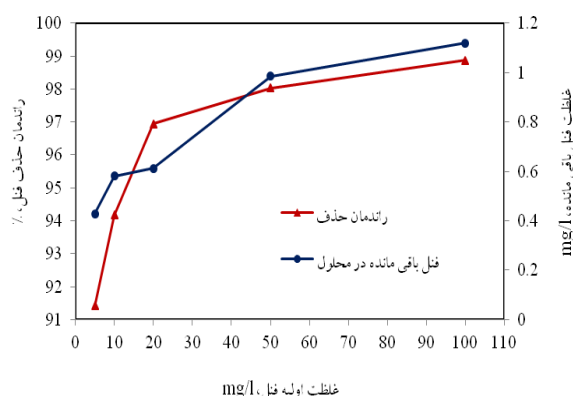
نمودار ۴- راندمان حذف فنل از آب شیر برداشت (نمونه واقعی) در غلظت‌های مختلف فنل (pH برابر ۵، غلظت منعقدکننده برابر ۰/۱ ml/L)
