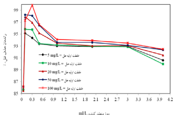
نمودار ۲- اثر غلظت اولیه منعقدکننده مورینگا پرگرینا بر حذف فنل در غلظت‌های مختلف (pH اولیه معادل ۵)
