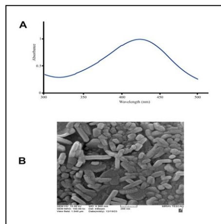
شکل ۳- طیف جذب uv-vis نانوذرات نقره سنتز شده با کرایزین (A) و آنالیز FESEM از نانوذرات نقره سنتز شده با کرایزین (B).
