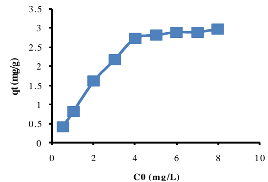
نمودار 12- ایزوترم جذبی لانگمویر مربوط به یون مس
