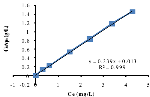
نمودار 13- ایزوترم جذبی فرنلیدج مربوط به یون مس
