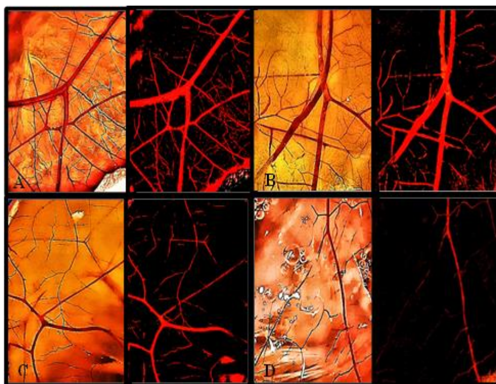
شکل ۲- تصاویر عکس‌برداری شده به وسیله استریو میکروسکوپ ۶۴× از پرده کوریوالانتوئیک (CAM) تحت تیمار با عصاره هیدروالکلی گیاه زرشک که میزان عروق به وسیله نرم‌افزار ImageJ آنالیز شده است: (A) گروه کنترل، B غلظت ۴۰ ماکروگرم بر میلی لیتر، C غلظت ۸۰ ماکروگرم بر میلی لیتر و D غلظت ۱۲۰ ماکروگرم بر میلی لیتر)
