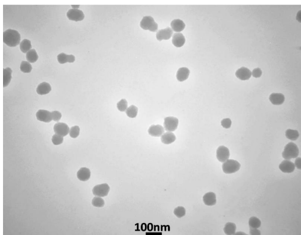
شکل ۱- مشخصه‌یابی نانوذرات سیلیکا آمینه با میکروسکوپ الکترونی عبوری
