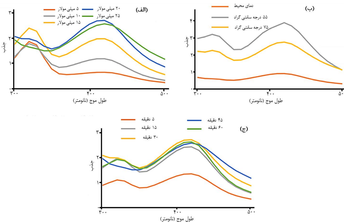
تصویر ۱- طیف UV-Vis نانوذرات نقره سنتز شده با عصاره دانه بارهنگ در غلظت‌های مختلف نیترات نقره (الف)، در دماهای مختلف (ب) و در بازه زمانی متفاوت (ج).
