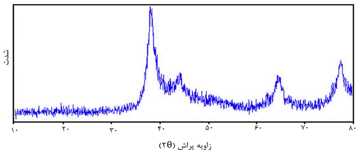
تصویر ۳- الگوی XRD مربوط به نانوذرات نقره سنتز شده با عصاره دانه بارهنگ
