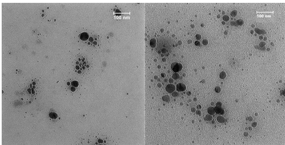
تصویر ۵- تصویر TEM مربوط به نانوذرات نقره سنتز شده با عصاره دانه بارهنگ
