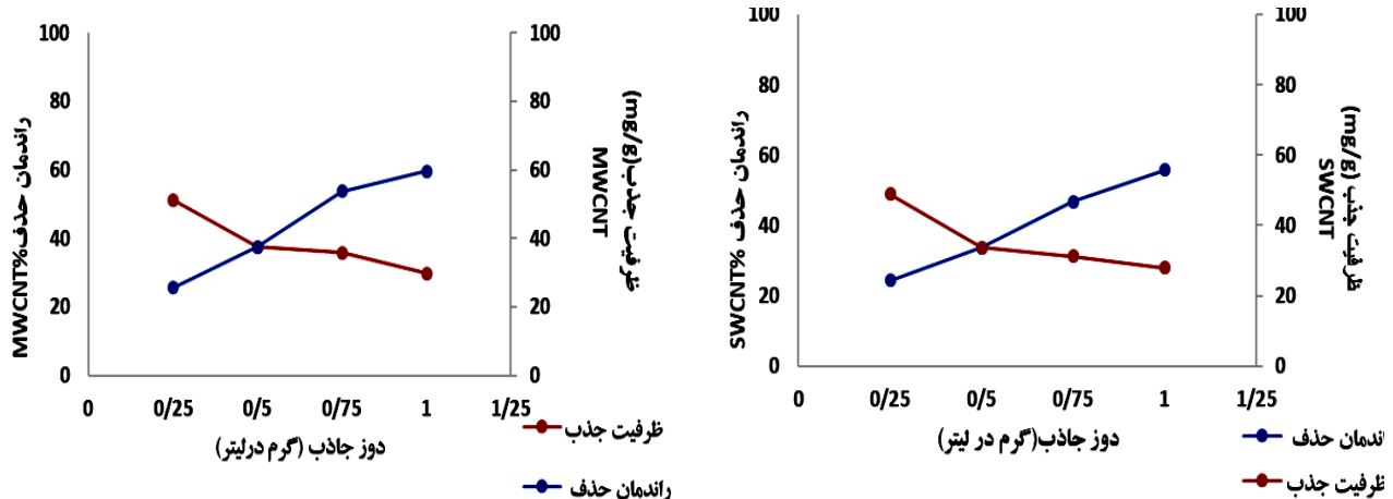
شکل ۵- بررسی دوز جاذب در کارایی حذف استامینوفن توسط نانولوله SWCNT (الف) و MWCNT (ب). [ 50 \text{ mg/L}^{-1} = غلظت اولیه استامینوفن، v=300 \text{ rpm} ، t=30 \text{ min} ، \text{pH}=7 ]
