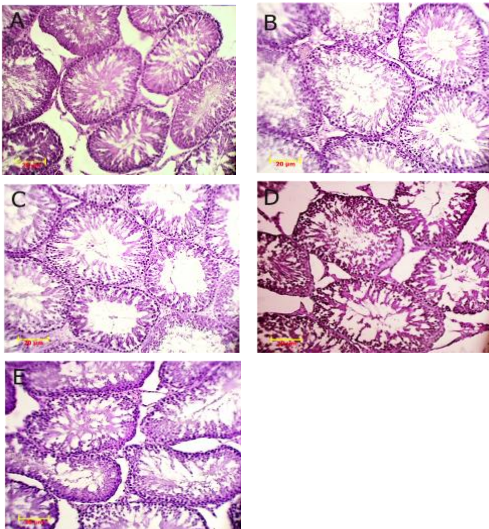
شکل ۱- تصاویر لوله‌های سمینفروس بافت بیضه گروه‌های مختلف با روش رنگ‌آمیزی هماتوکسیلین و ائوزین (H&E): A: گروه کنترل، B: گروه شاهد، C: گروه دارچین، D: گروه صدا و E: گروه صدا+دارچین (Scale bar, 20 µm)
