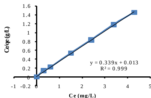
نمودار 128- ایزوترم جذبی لانگمویر مربوط به یون مس
