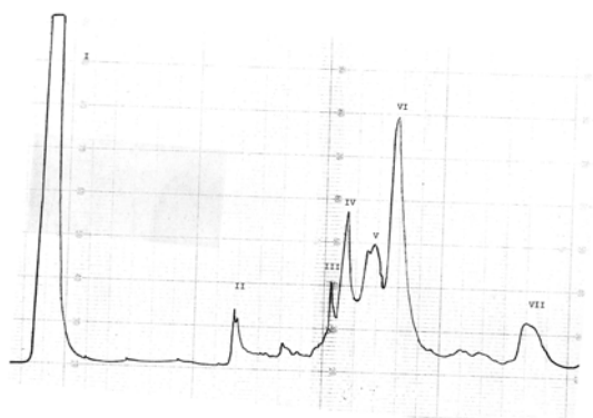
شکل ۱- کروماتوگرام رسوبات جدا شده از لاتکس (با استفاده از روش جداسازی با نمک) روی ستون Mono-S با گرادیان غلظت و \text{pH} بافر فسفات
