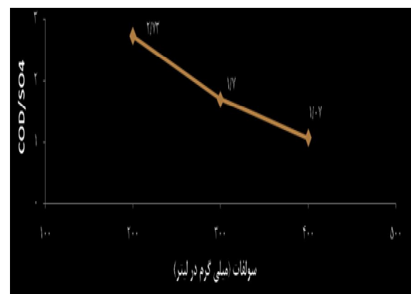
نمودار 1- تأثیر افزایش سولفات بر نسبت COD به SO_4 در پساب خروجی پیلوت برکه تثبیت بی‌هوازی
