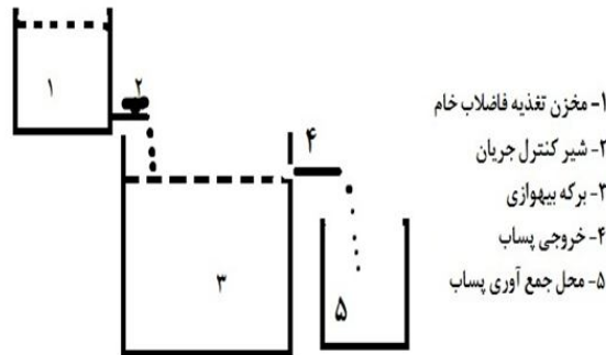
شکل 1- شماتیک برکه تثبیت بی‌هوازی با ابعاد 0/4 \times 0/4 \times 1 متر در مقیاس 1:250 و زمان ماند هیدرولیکی 7/5 روز
