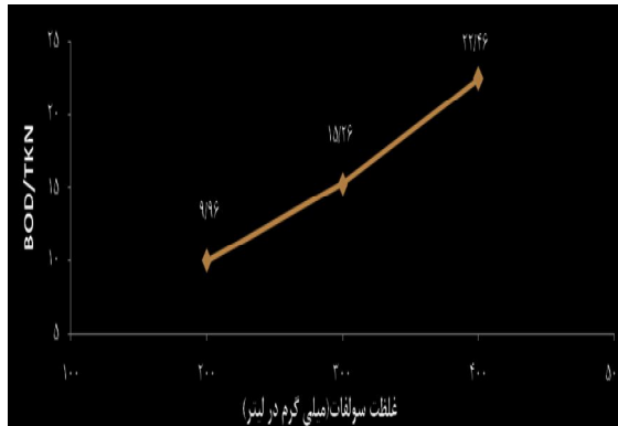
نمودار 2- تأثیر افزایش سولفات بر نسبت BOD به TKN در پساب خروجی پیلوت برکه تثبیت بی‌هوازی
