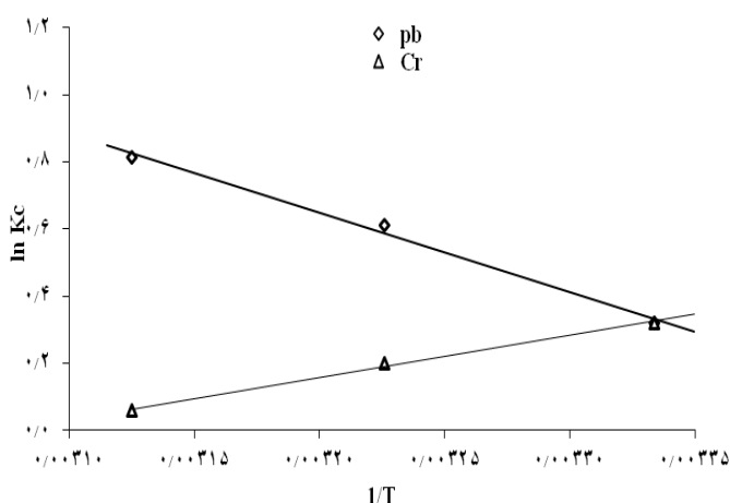
نمودار 9- رسم خطی \ln K_c در برابر 1/T برای جذب سطحی کروم و سرب توسط نانوذرآت گرافن اکساید
