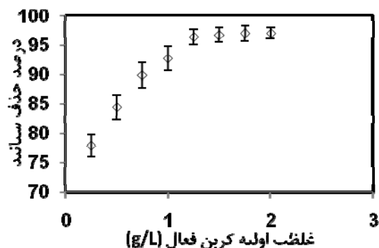
شکل ۳- تأثیر دوز جاذب بر راندمان حذف سیانید (pH اولیه محلول ۹، غلظت اولیه سیانید ۱۰۰ mg/L، زمان تماس ۴۰ دقیقه)
