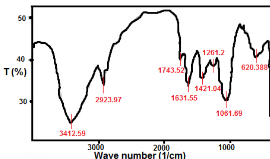
شکل ۱- طول موج FTIR کربن فعال اصلاح شده با هیدروکسید سدیم در طول موج‌های 4000 \text{ cm}^{-1} تا 450 \text{ cm}^{-1}
