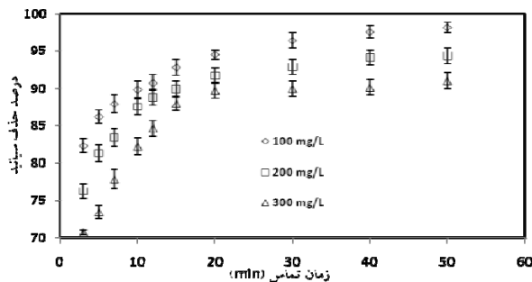
شکل ۴- تأثیر غلظت‌های اولیه سیانید بر درصد حذف آن توسط کربن فعال اصلاح‌شده با هیدرواکسید سدیم (pH اولیه محلول ۹، دوز جاذب ۱/۲۵ g/L، زمان تماس ۶۰ دقیقه)
