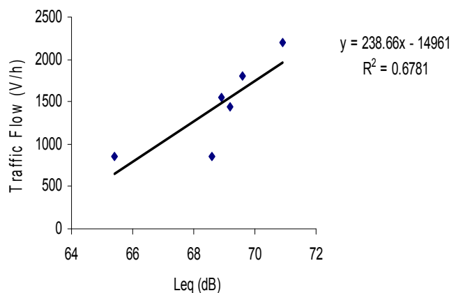
نمودار ۱- رابطه همبستگی میان تغییرات میانگین تراز صوت و فلوی ترافیک در ایستگاه خیابان طالقانی. آزمون ضریب همبستگی پیرسون، رابطه معنی‌دار میان تغییرات میانگین تراز صوت و حجم ترافیک عبوری را نشان داد ( r = 0.82 , P < 0.05 ).
