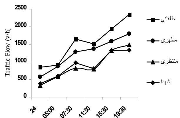
نمودار ۳- فلوی ترافیک در ساعات مختلف روزهای کاری هفته در ایستگاه‌های مورد بررسی
