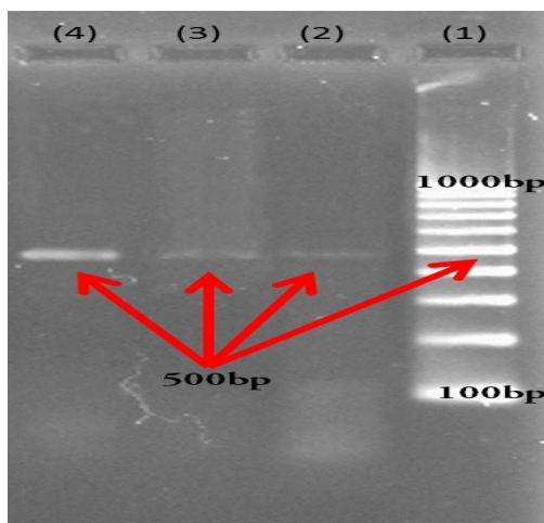
شکل ۵- نتایج حاصل از RT-PCR و متعاقباً PCR. الکتروفورز محصول RT-PCR و PCR بر روی سلول حاوی وکتور در حضور و عدم حضور siRNA اختصاصی بر روی ژل آگارز ۱٪/۵ (۱) لدر ۱۰۰۰bp (۲) PCR از cDNA سلول حاوی وکتور در مواجهه با siRNA2 از کاهش میزان mRNA حکایت دارد. (۳) PCR از cDNA سلول حاوی وکتور در مواجهه با siRNA1 از کاهش میزان mRNA حکایت دارد. (۴) PCR از cDNA سلول حاوی وکتور در عدم حضور siRNA.
