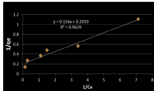
شکل 9- ایزوترم جذب کادمیوم توسط نانوذرات زیستی نقره بر اساس مدل لانگمویر
