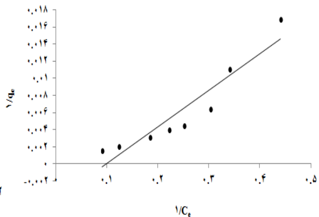
نمودار ۶- ایزوترم جذب لانگمویر برای جذب سطحی رنگ راکتیو قرمز ۱۹۸ بر روی خاکستر پوسته میوه پسته
