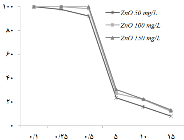
شکل ۴- میزان حذف کروم شش ظرفیتی در غلظت‌های مختلف کروم و نانوذره اکسید روی (زمان تابش ۱۵ دقیقه)
